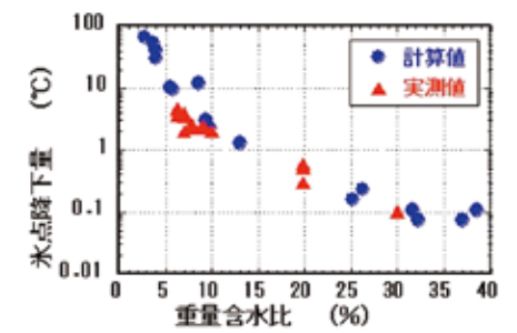
図1 荒木田土の氷点降下量と含水比の関係
